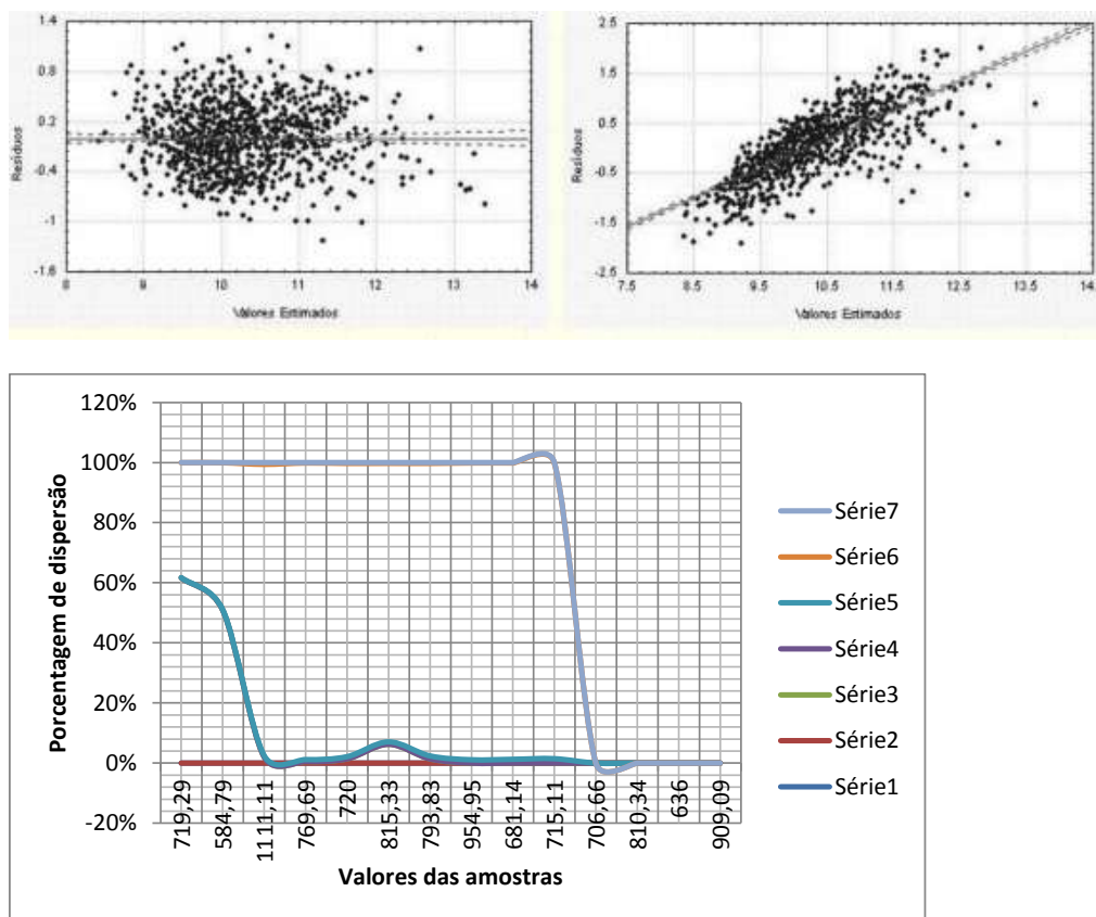
Figura 64: Gráfico de homocedasticidade.
