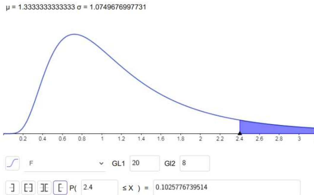
Figura 67: Distribuição F de Snedecor. Obtido junto ao Software GEOGEBRA. A Área branca representa a área de aceitação dos dados amostrais.
